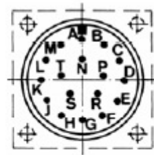
MS 3102 A 20-29 P (17 PIN) MIL
