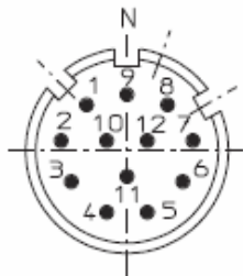
12-poliger Stecker
