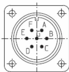
7-poliger MIL-Stecker
