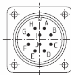
10-poliger MIL-Stecker
