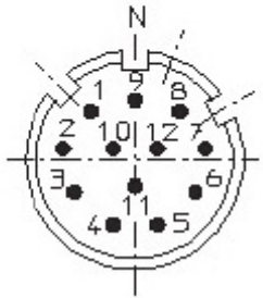
Ansicht auf Steckseite Stiftkontakteinsatz: 12-poliger Stecker
